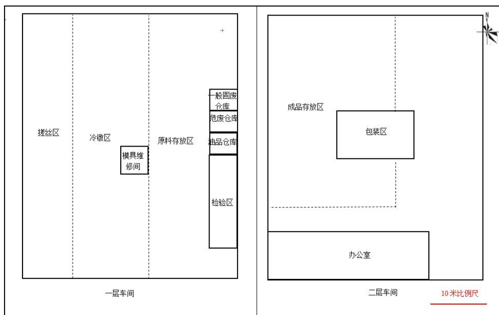
图 2-1 本项目平面布置图
