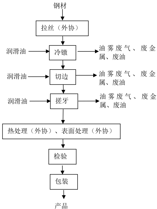
图 2-2 生产工艺流程及产污环节图
