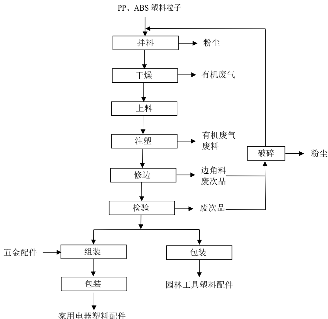
图 3-5 本项目家用电器塑料配件和园林工具塑料配件生产工艺流程及产污环节图
