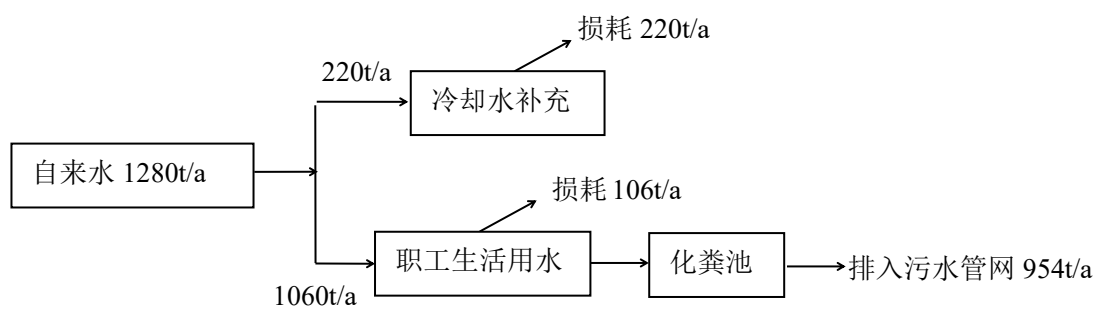
图 3-4 水平衡图（单位 t/a）
